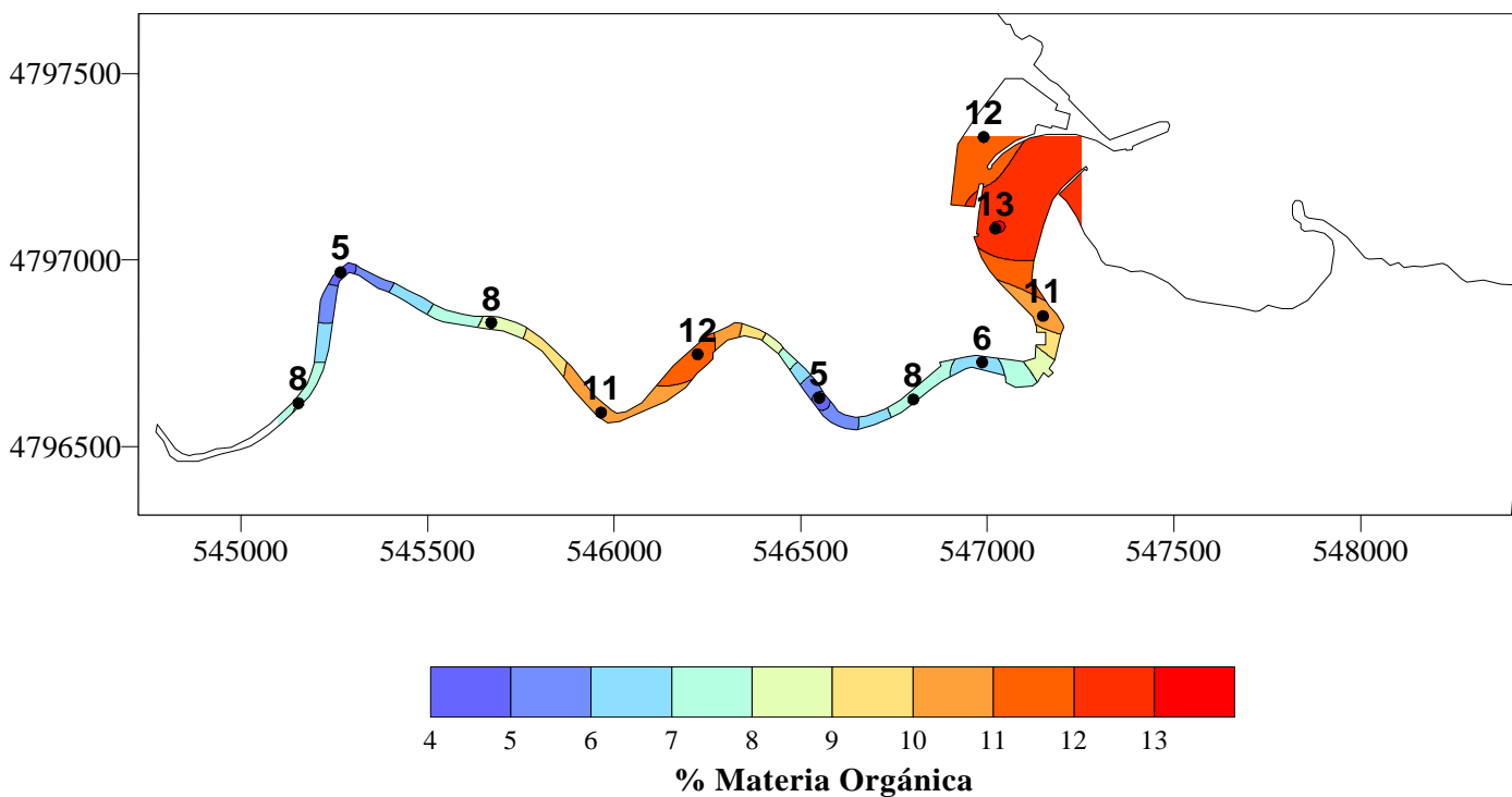
Figura 7.2. Distribución del contenido en limos y de materia orgánica en los sedimentos del estuario del Artibai.
