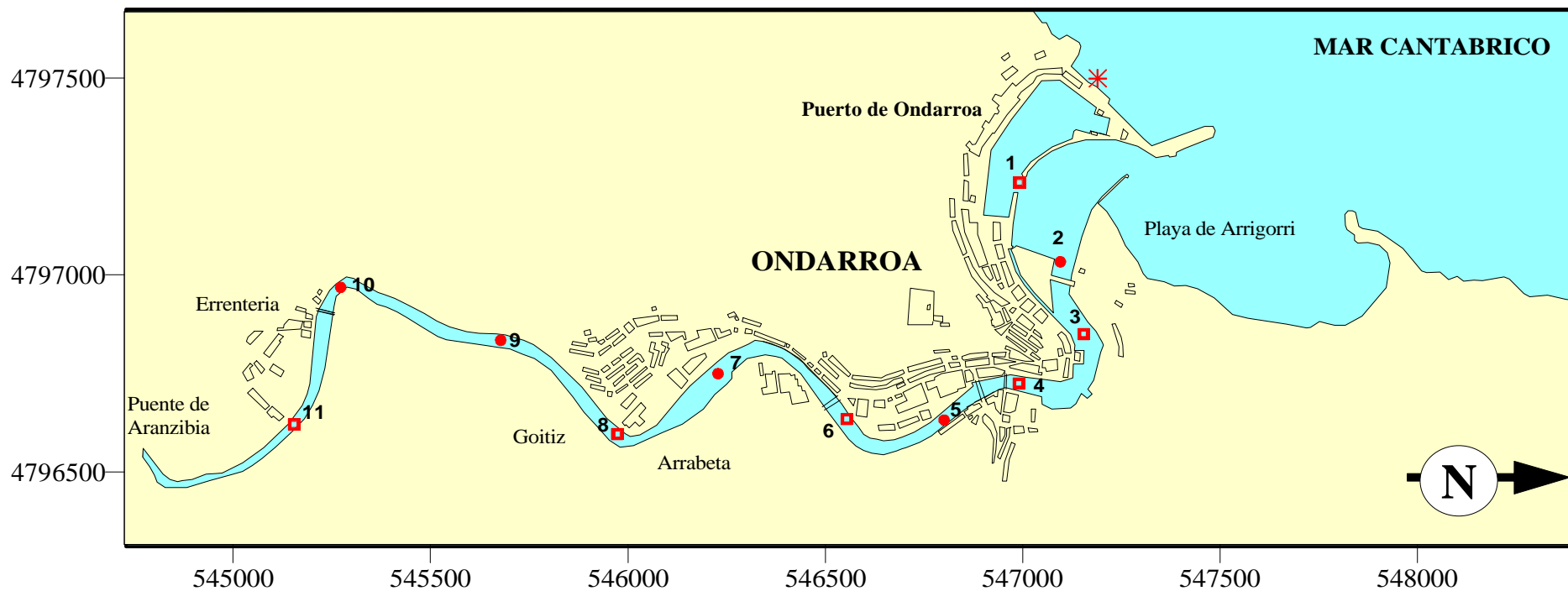
Figura 7.1. Situación de las estaciones de muestreo en el estuario del Artibai.
