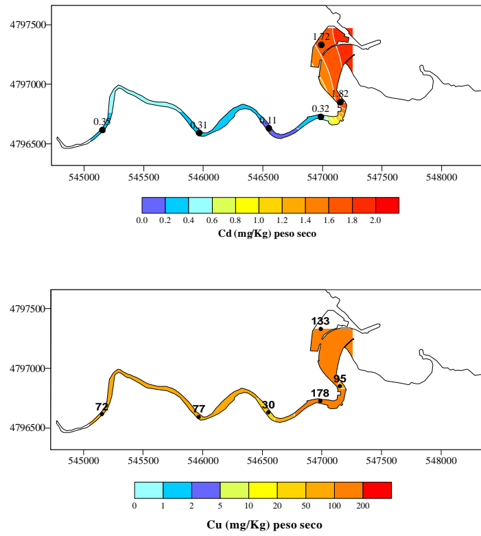
Figura 7.9. Distribución del contenido de cadmio y cobre en los sedimentos del estuario del Artibai.
