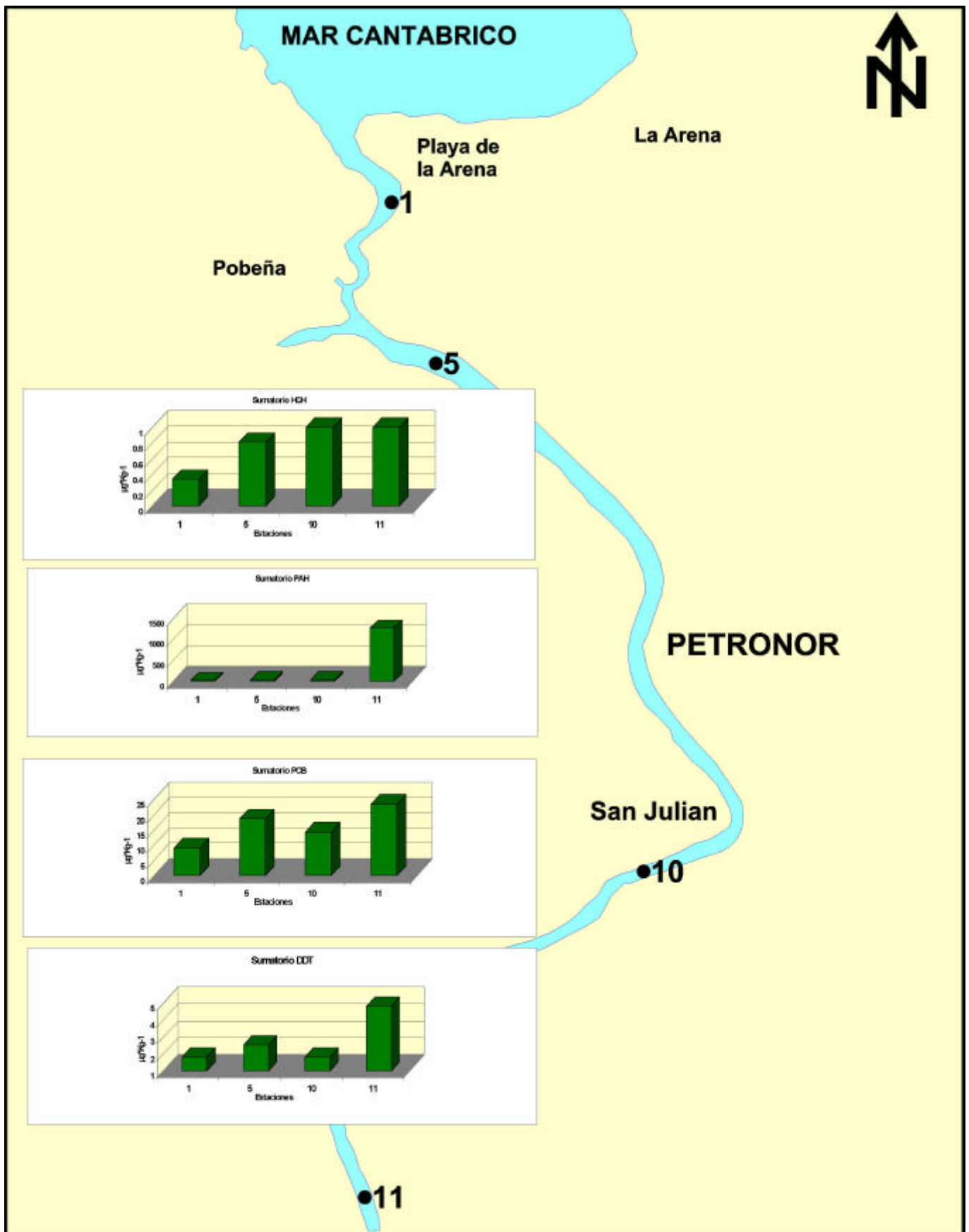
Figura 6.6 Distribución de los compuestos orgánicos en los sedimentos del estuario del Barbadún.
