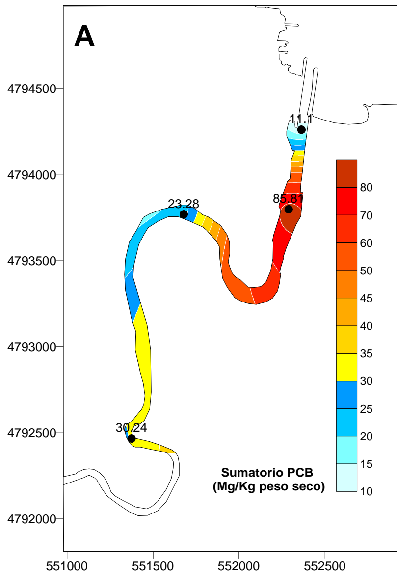
Figura 7.10 : Distribución del sumatorio de los valores de PCB (a) y del sumatorio de los valores de PAH (b) en los sedimentos del río Deba.
