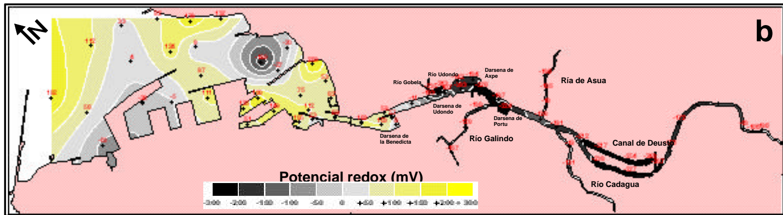
Figura 5.3. Relación C/N (a) y potencial redox (b) en los sedimentos del estuario del Nerbioi.
