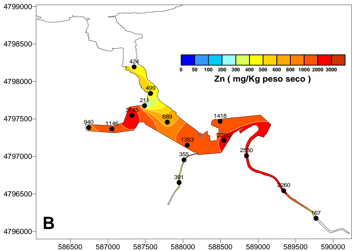
Figura 5.7 : Distribución de los valores de hierro (a) y zinc (b) en los sedimentos del río Oiartzun y de la bahía de Pasaia.
