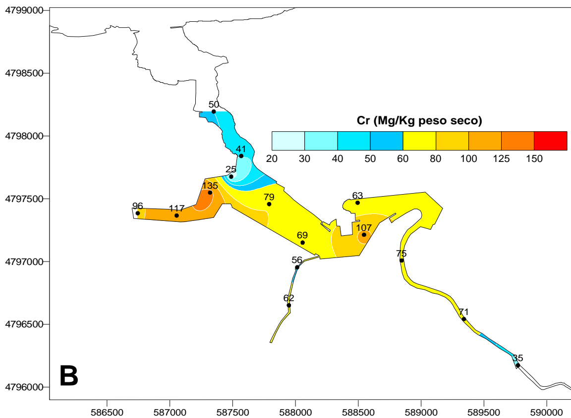
Figura 5.8 : Distribución de los valores de níquel (a) y cromo (b) en los sedimentos del río Oiartzun y de la bahía de Pasaia.
