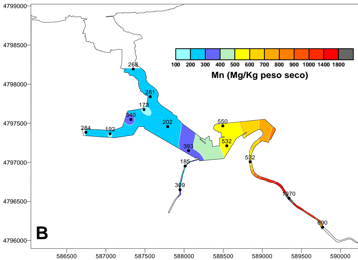
Figura 5.9 : Distribución de los valores de plomo (a) y manganeso (b) en los sedimentos del río Oiartzun y de la bahía de Pasaia.
